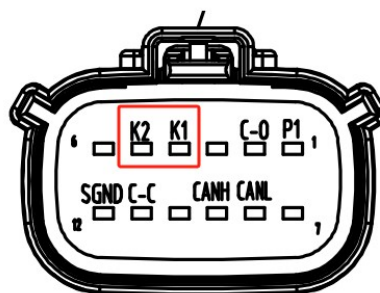
CAN节点
